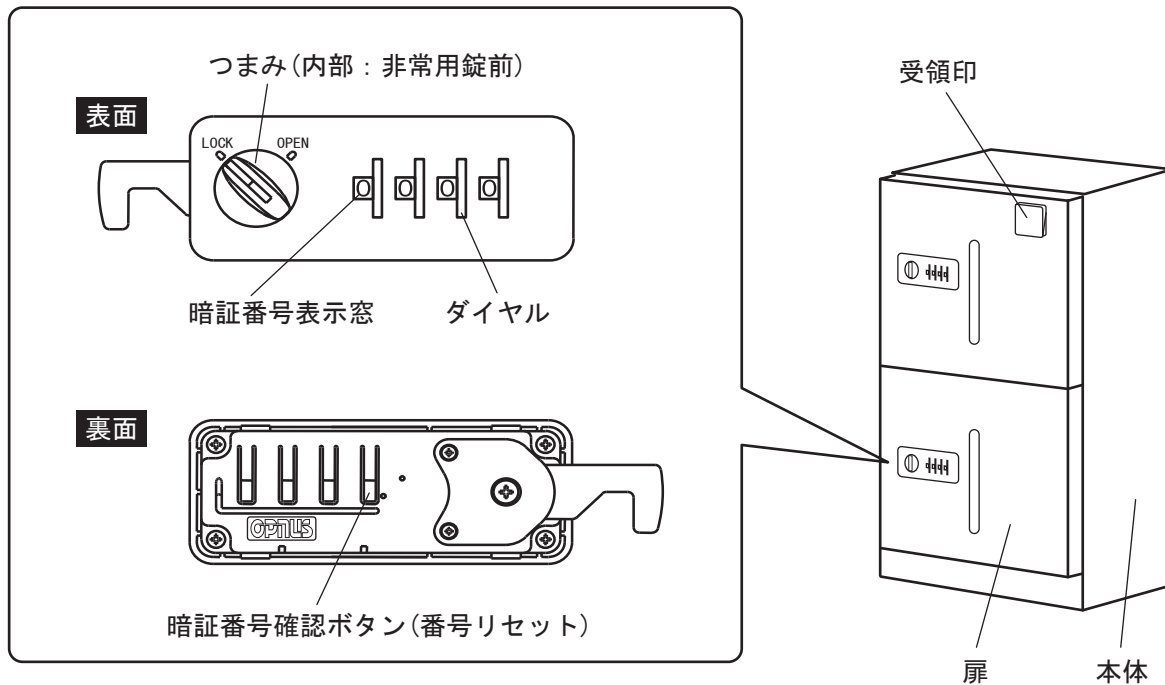
錠前詳細図
