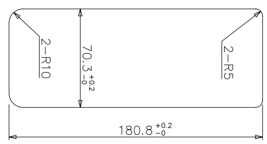
取付穴参考図 (t0.7~1.0)
