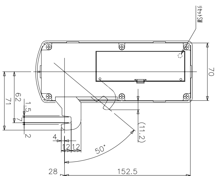
取付穴参考図 (t0.7~1.0)
